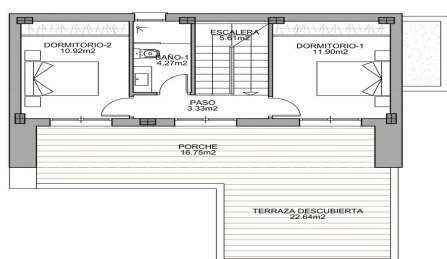
PLANTA PRIMERA
