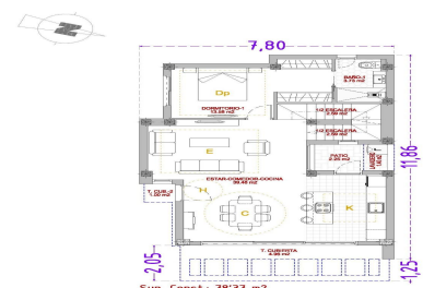
TIPO-05 VIVIENDAS Nº: 18 PL/ BAJA.
